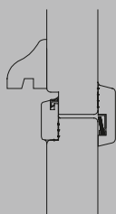
doorsnede duodeling
